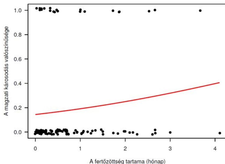
I/75. ábra. A terhességi szövődmények valószínűsége a magzat Borrelia expozíciós időtartamának a függvényében. A 0 érték körül szétszórott pontokkal jelöltük az eseménymentes, az 1 körüliekkel a szövődményes eseteket. (Solymosi Norbert ábrája.)
