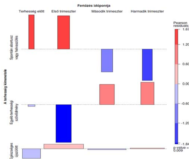
I/74. ábra. A terhesség kimenetele és a fertőzés időpontja közötti összefüggés. A fertőzés időpontját az 1. klinikai tünet megjelenésétől számítottam. Az asszociációs ábrán a megfigyelt gyakoriságoknak a véletlenszerű eloszlástól való eltérését mutatják az oszlopok. Az oszlopok magassága (Pearson reziduális) az eltérés mértékével, szélessége pedig a várható gyakorisággal arányos. Az alaponál (szaggatott vízszintes vonal) való függőleges eltérés iránya jelzi, hogy a megfigyelt gyakoriság a véletlenszerű eloszlás esetén várható gyakoriságnál nagyobb (felfelé) vagy kisebb (lefelé). (Solymosi Norbert ábrája.)
